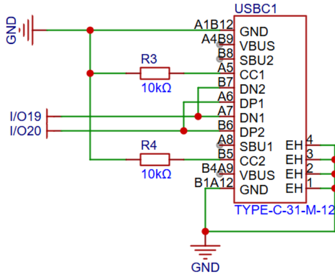
Hình 3.7: Sơ đồ mạch giao tiếp USB Type-C
