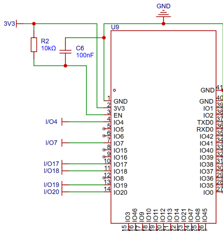
Hình 3.5: Sơ đồ kết nối vi xử lí ESP32-S3
